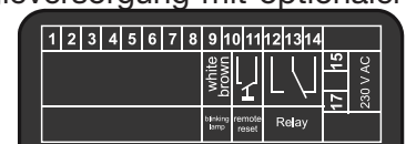
Bild 1 - Anschlüsse EKL8000
