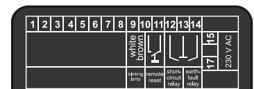
Bild 2 - Anschlüsse EKL8001
