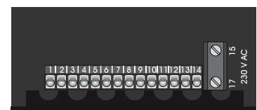
Bild 3 - Anschlüsse
